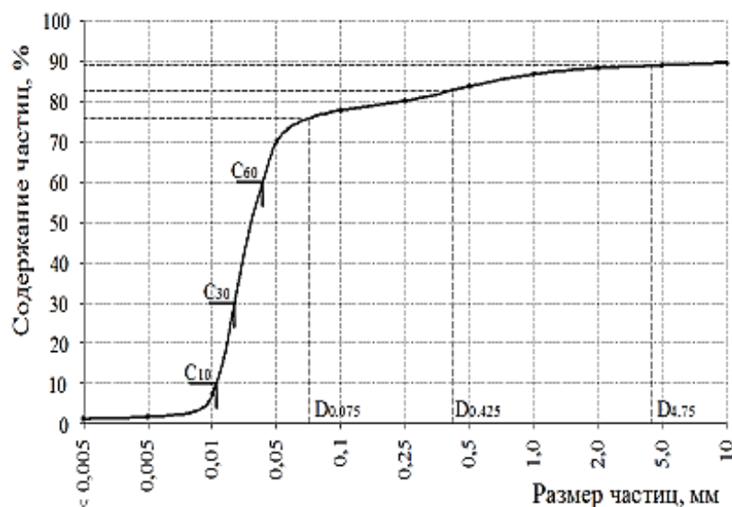
Рисунок Е.1 - Кумулятивная кривая гранулометрического состава
