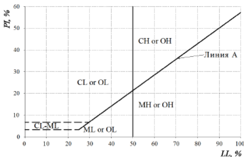
Рисунок Е.2 - График пластичности грунтов (Plasticity Chart)
